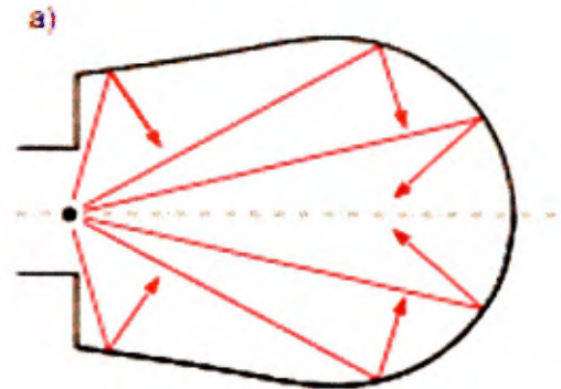
Sala en forma de herradura. Generación de reflexiones laterales.
