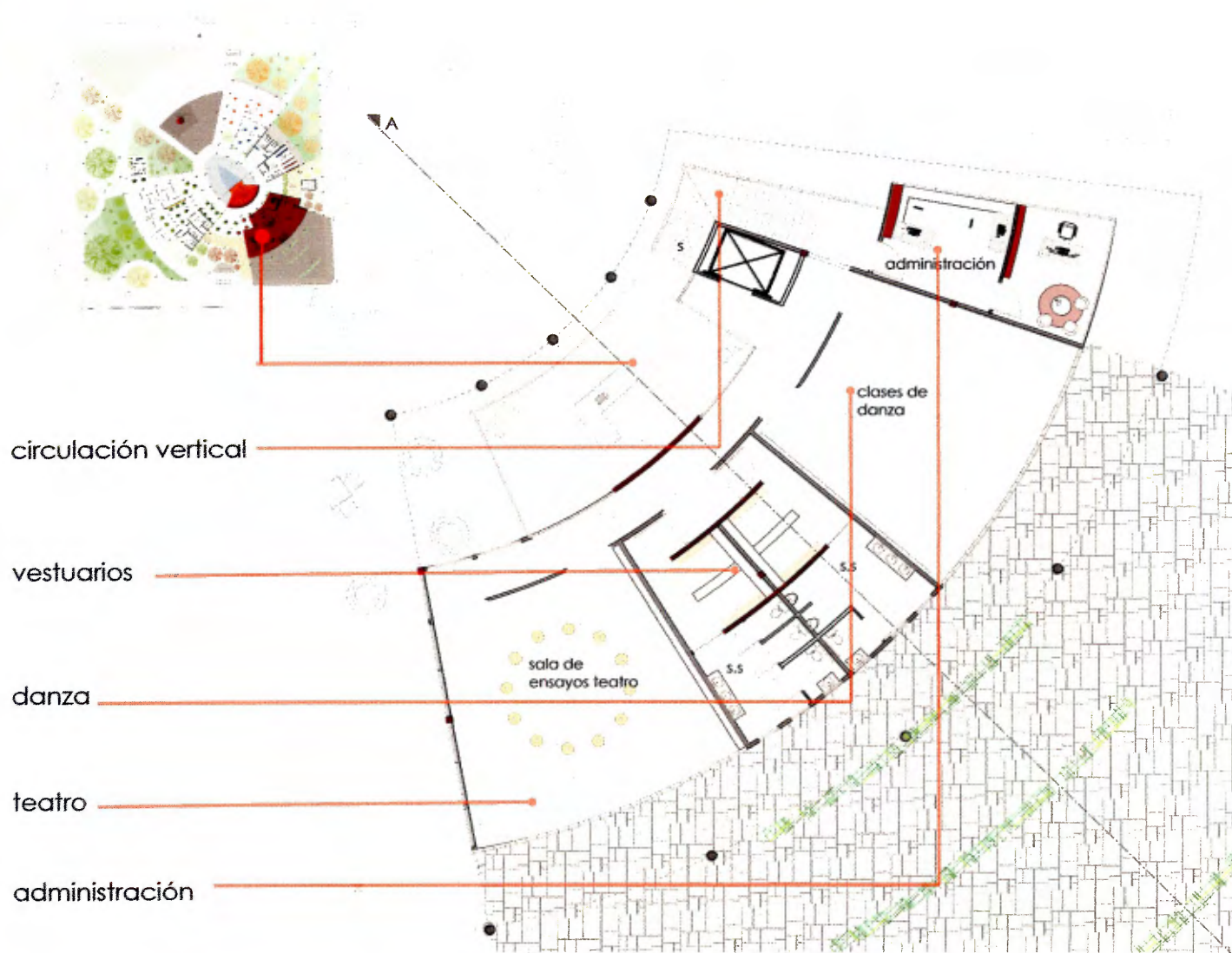
Planta nivel +3.50 m Danza y Teatro
