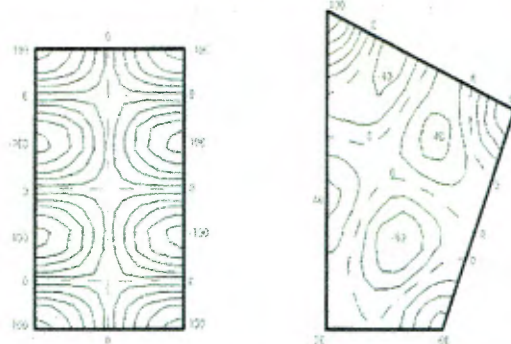
Distribución de módulos en cuartos con formas diferentes
