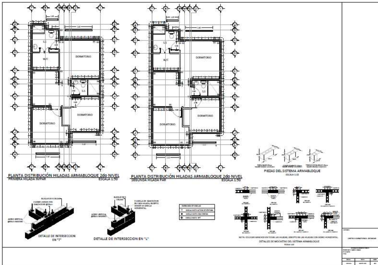
Figura 47. Planta de distribución de paredes Armabloque.
