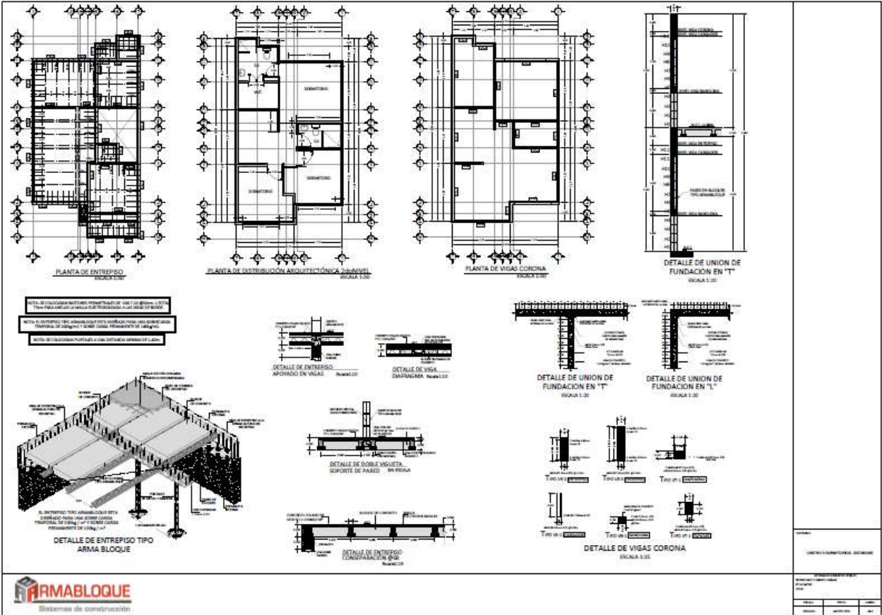
Figura 46. Detalle estructural de vigas
