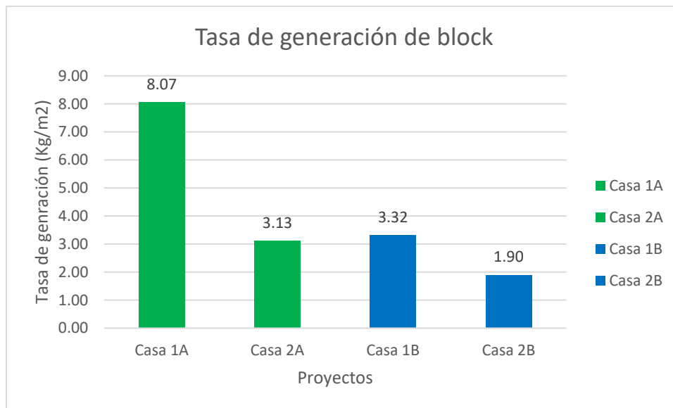
Figura 41. Tasa de generación de bloques de concreto (Kg/m 2 ).
