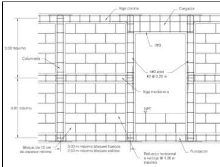
Figura 4. Elevación de pared mampostería confinada
