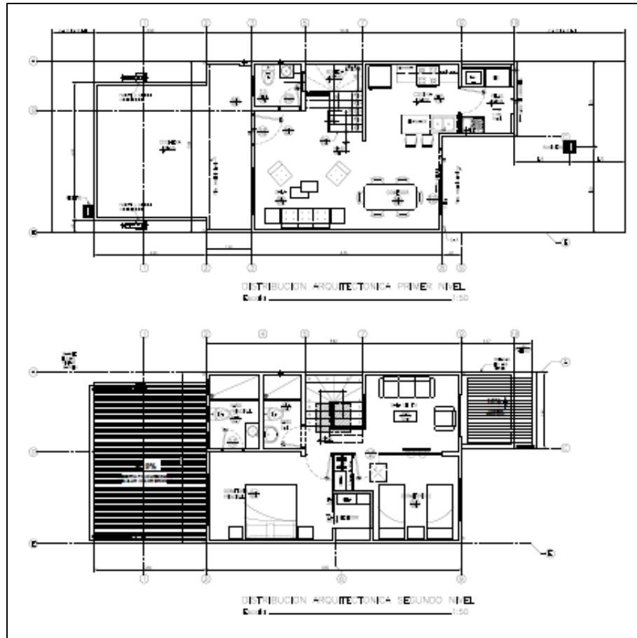
Figura 11. Distribución arquitectónica de los proyectos 1B y 2B.
