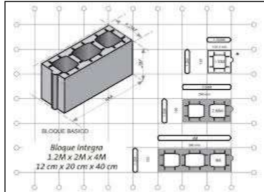
Figura 5. Detalle de bolque integra PC
