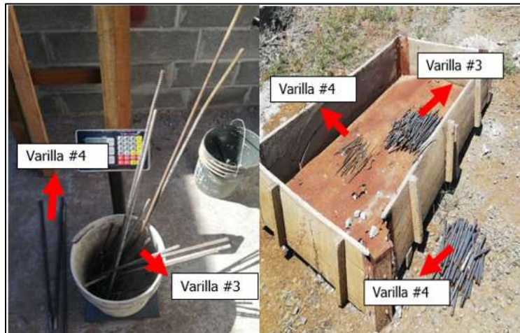
Figura 29. Muestras de varillas en los proyectos 1A y 1B.
