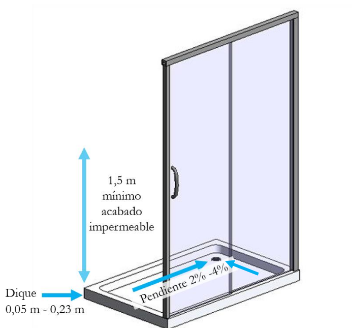
Figura 37. Requisitos para las duchas Fuente: Elaboración propia, 2021
