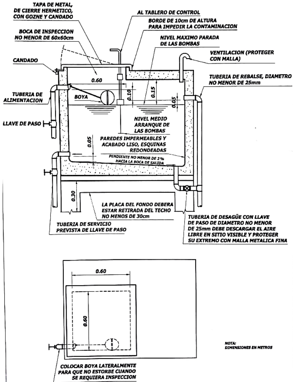
Figura 1. Tanque elevado de almacenamiento de agua Fuente: CIHSE, 2017
