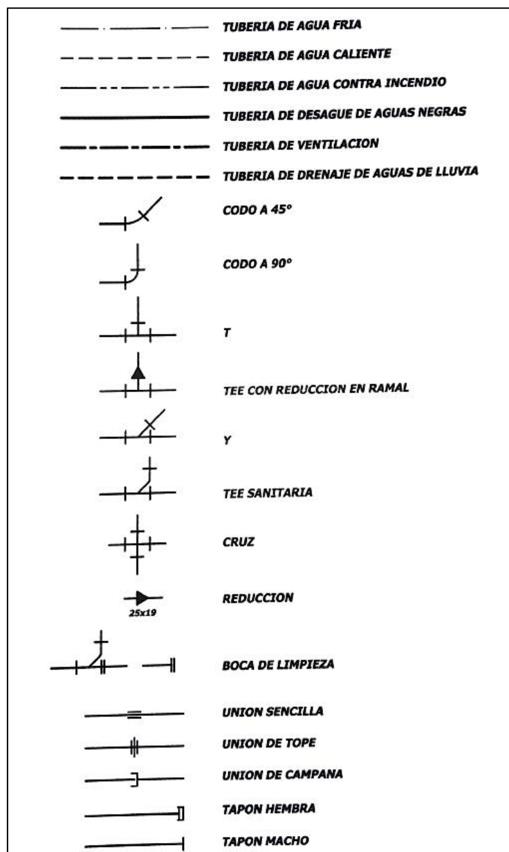
Figura 62. Primera parte de símbolos gráficos de instalaciones sanitarias Fuente: CIHSE, 2017
