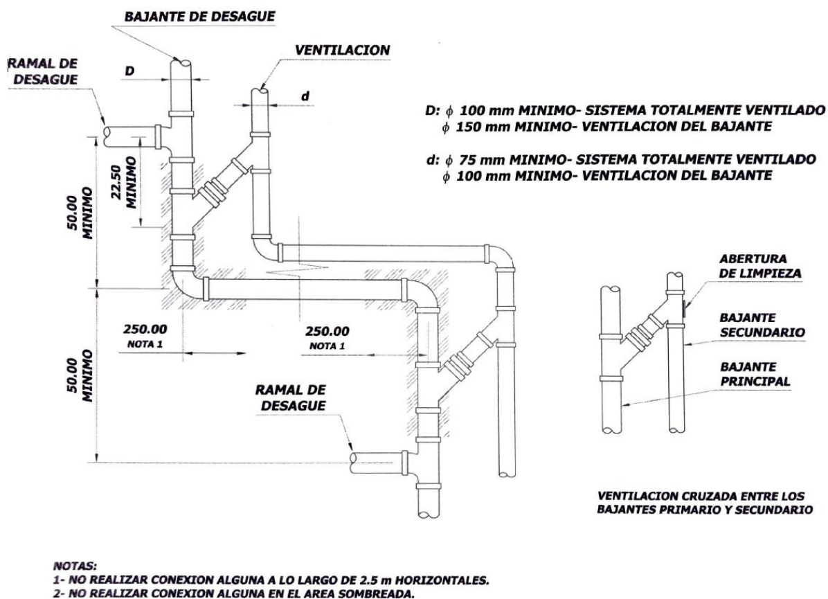
Figura 51. Ventilación del bajante de aguas residuales Fuente: CIHSE, 2017
