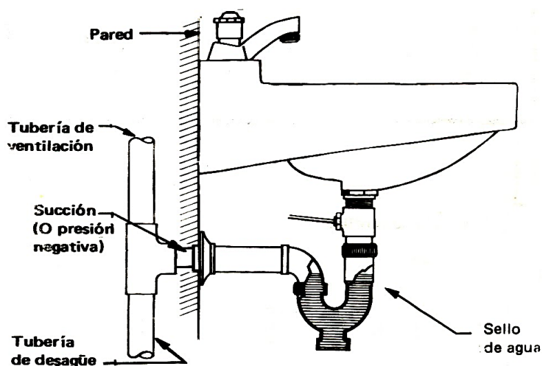
Figura 32. Sello de agua de lavatorio Fuente: Google, 2021
