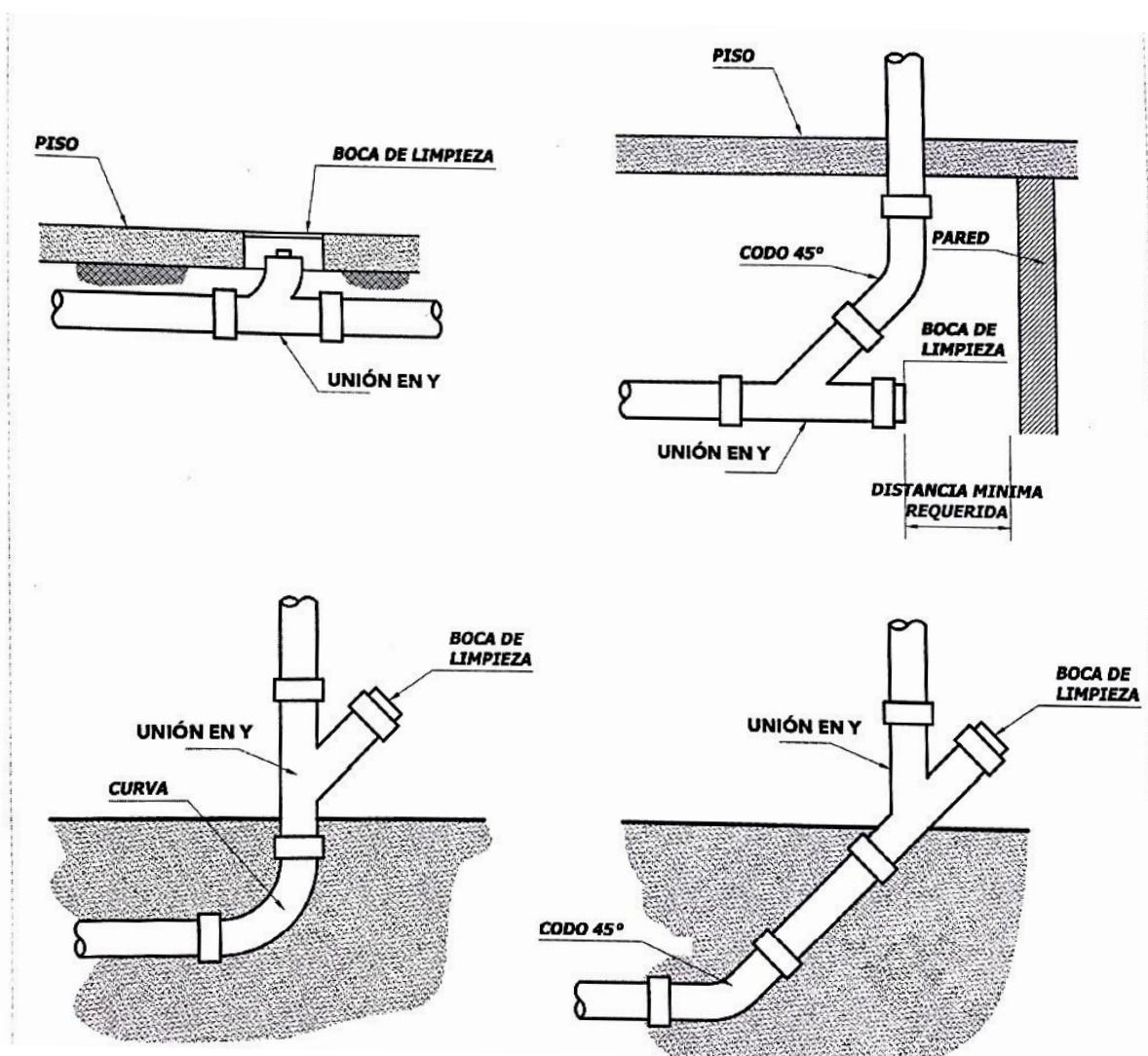
Figura 41. Bocas de limpieza Fuente: CIHSE, 2017
