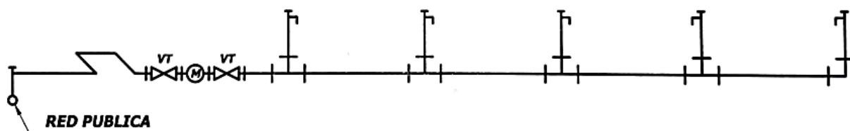
Figura 21. Esquema de alimentación de agua potable en sistema directo Fuente: CIHSE, 2017
