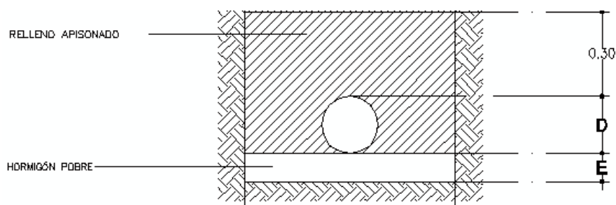
Figura 39. Zanja para tubería sanitaria Fuente: Google, 2021
