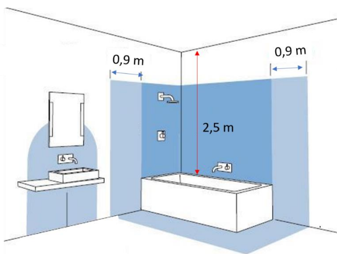
Figura 16. Distancias prohibidas para luminarias en baños Fuente: Elaboración propia, 2021
