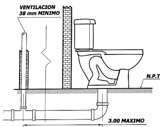
Figura 35. Distancia máxima entre la tubería de ventilación y la salida del inodoro Fuente: CIHSE, 2017
