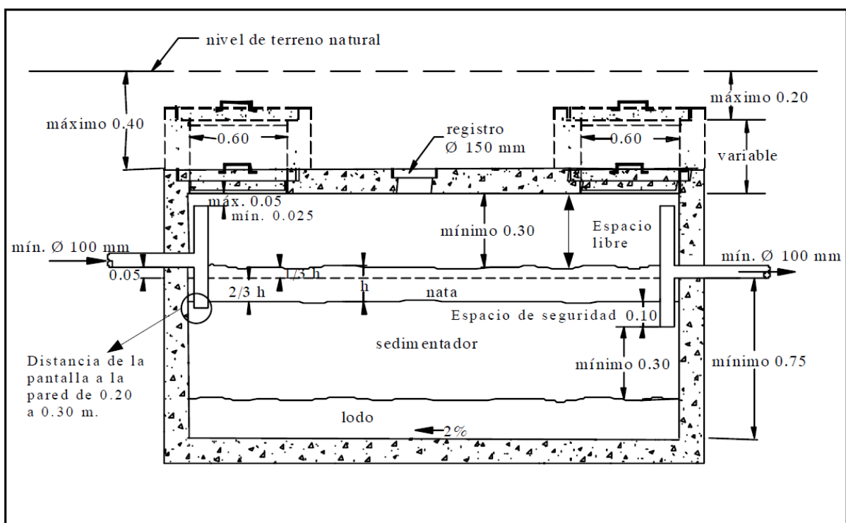
Figura 46. Ejemplo de tanque séptico Fuente: OPS, CEPIS y UNATSABAR
