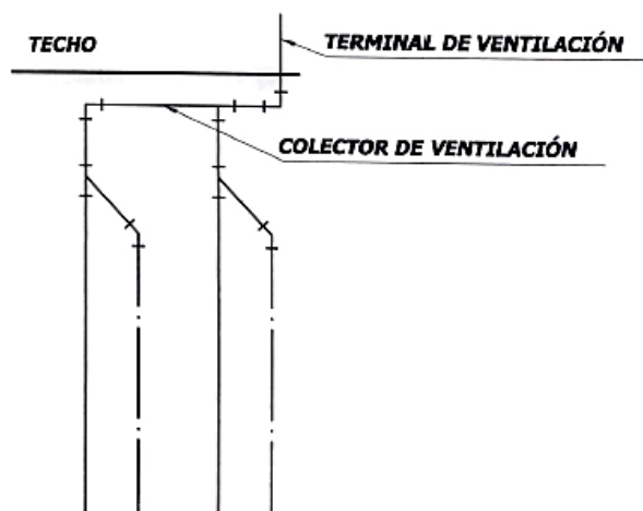
Figura 48. Conexión del extremo superior al bajante de aguas residuales Fuente: CIHSE, 2017
