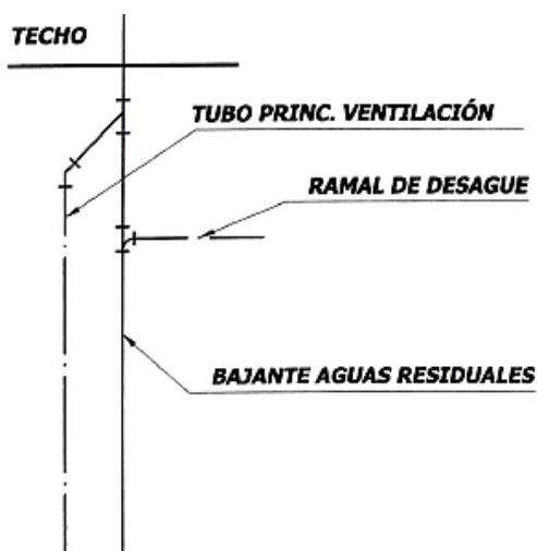
Figura 48. Conexión del extremo superior al bajante de aguas residuales Fuente: CIHSE, 2017
