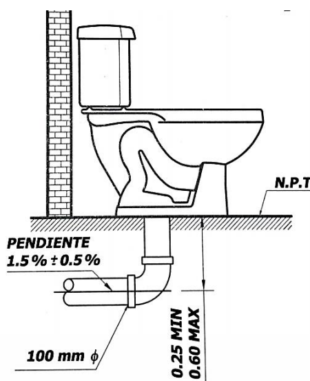
Figura 36. Distancia entre el codo sanitario y el nivel del piso Fuente: CIHSE, 2017
