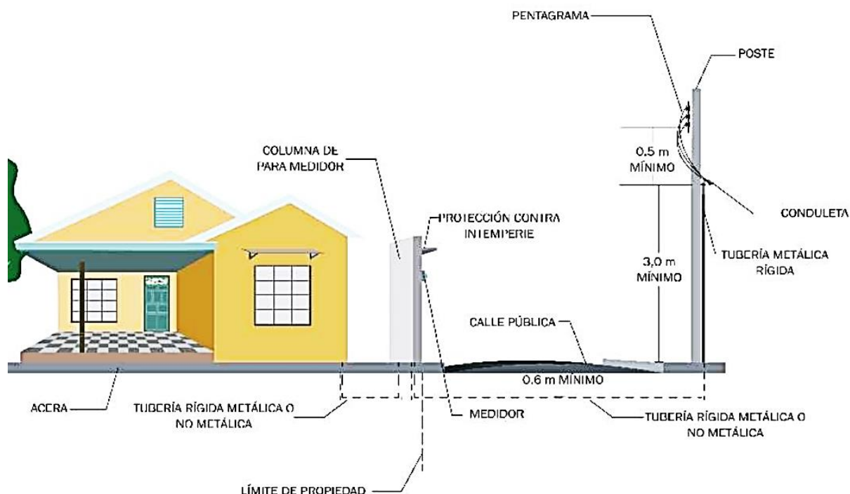
Figura 10. Acometida subterránea con columna de concreto para medidor Fuente: ARESEP, 2015
