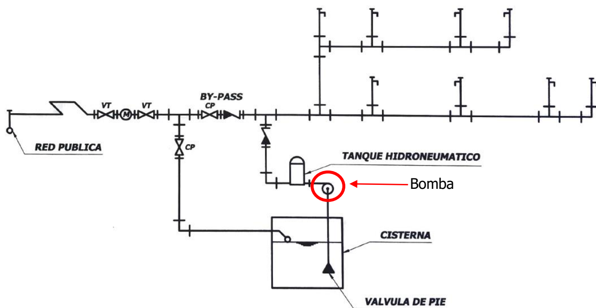
Figura 28. Esquema de sistema indirecto con bomba y tanque hidroneumático
