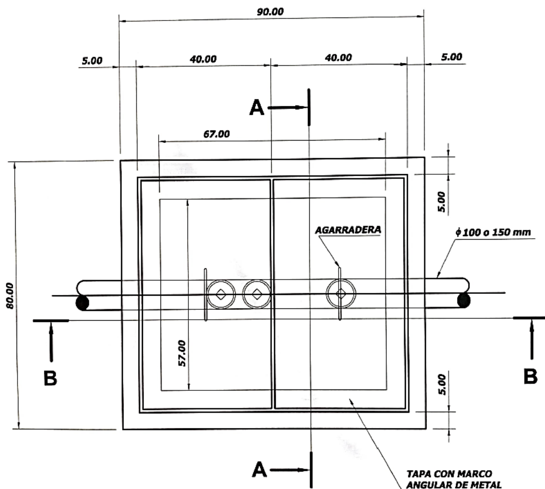
Figura 42. Vista superior de caja de registro domiciliar con sifón Fuente: CIHSE, 2017
