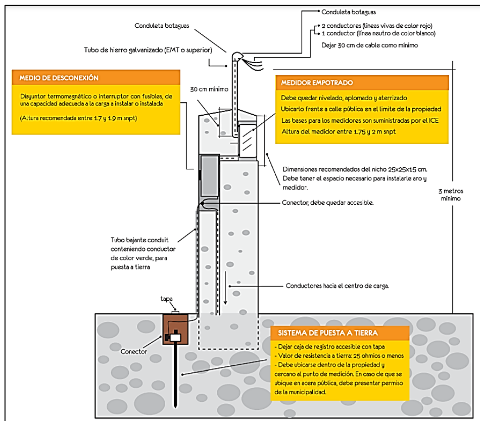
Figura 7. Columna con medio de desconexión y medidor empotrado
