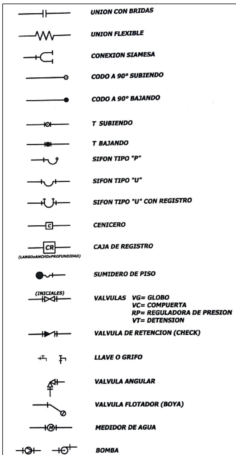
Figura 63. Segunda parte de símbolos gráficos de instalaciones sanitarias Fuente: CIHSE, 2017
