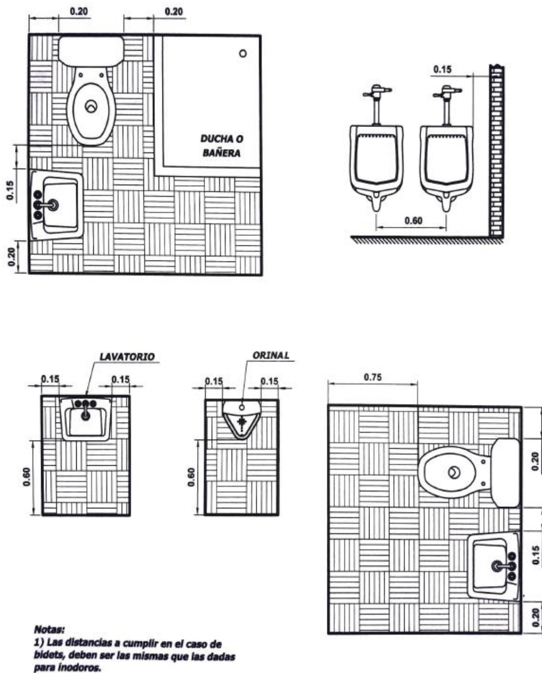
Figura 3. Dimensiones mínimas para la instalación de piezas sanitarias Fuente: CIHSE, 2017
