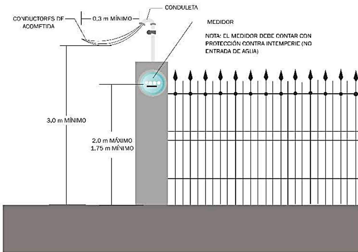
Figura 8. Medidor en el límite de la propiedad Fuente: ARESEP, 2015
