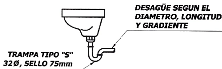
Figura 53. Sello de agua de ventilación de bajante único
