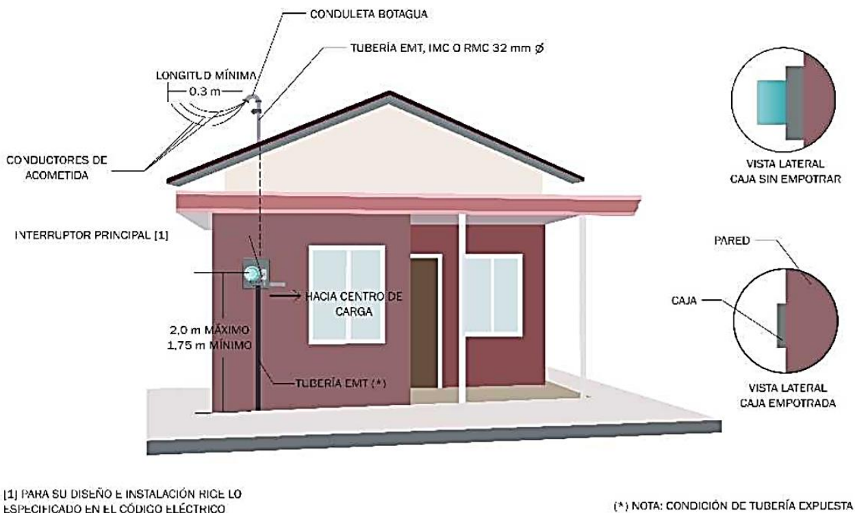
Figura 5. Caso de instalación de medidor en caja sobre pared Fuente: ARESEP, 2015
