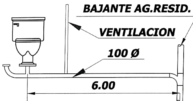
Figura 54. Inodoros con sistema de bajante único Fuente: CIHSE, 2017
