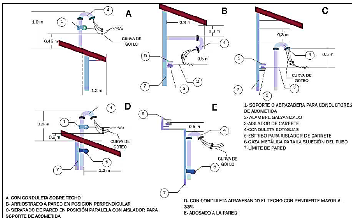
Figura 6. Separaciones mínimas según el caso de conduleta
