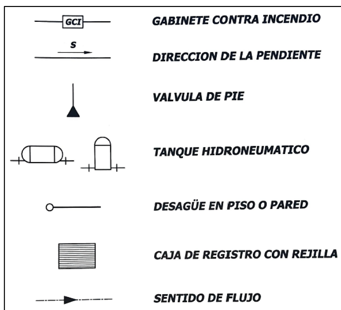
Figura 64. Tercera parte símbolos gráficos de instalaciones sanitarias Fuente: CIHSE, 2017
