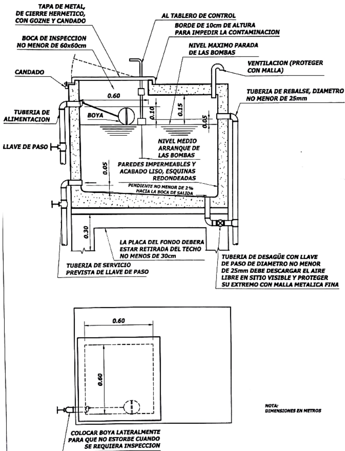
Figura 25. Tanque elevado de almacenamiento de agua
