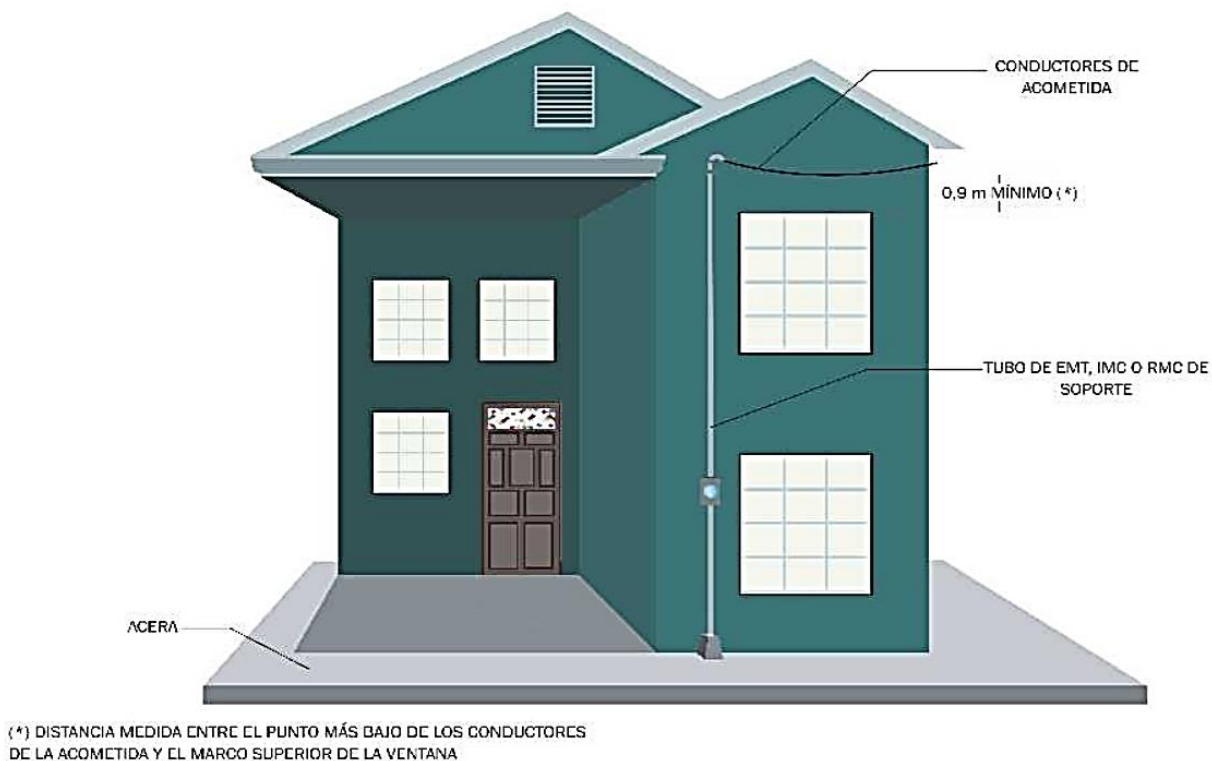
Figura 4. Separación de conductores de acometida de aberturas
