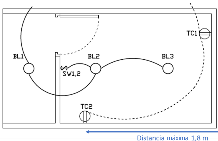
Figura 13. Distancia mínima horizontal para tomacorrientes Fuente: Elaboración propia, 2021
