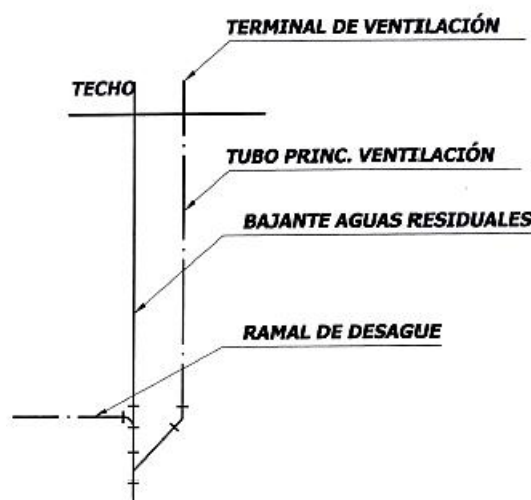
Figura 47. Conexión de la tubería principal de ventilación con el bajante de aguas residuales Fuente: CIHSE, 2017
