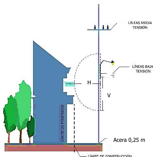
Figura 2. Distancias mínimas entre conductores de distribución y edificios Fuente: ARESEP, 2015
