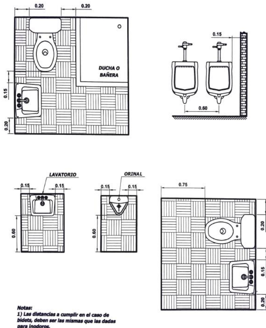
Figura 38. Dimensiones mínimas para la instalación de piezas sanitarias Fuente: CIHSE, 2017
