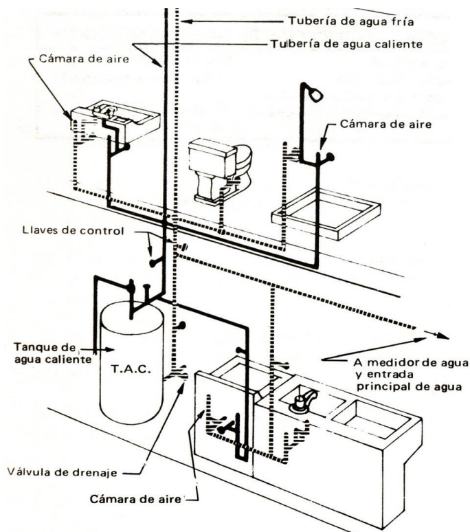
Figura 23. Cámaras de aire
