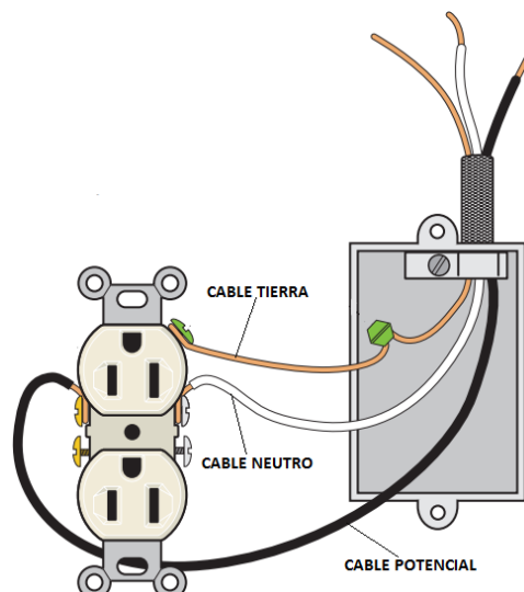
Figura 12. Partes de un tomacorriente Fuente: Google, 2015
