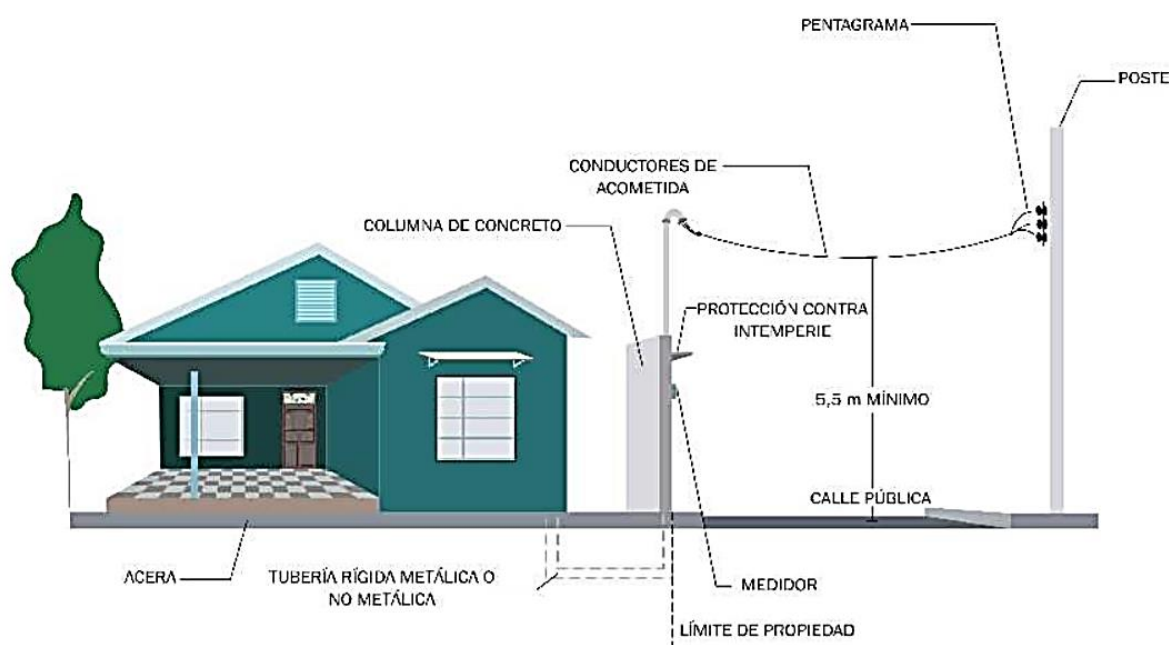
Figura 3. Separaciones mínimas para conductores de acometida aérea con respecto al centro de calle pública
