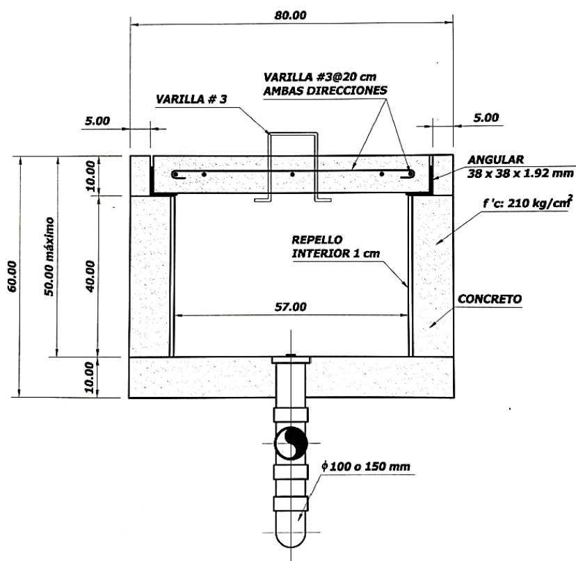
Figura 43. Sección A-A de caja de registro domiciliario con sifón Fuente: CIHSE, 2017
