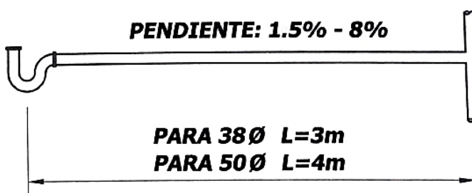
Figura 55. Sistemas de bajante único para pilas, tinajas, duchas y fregaderos Fuente: CIHSE, 2017
