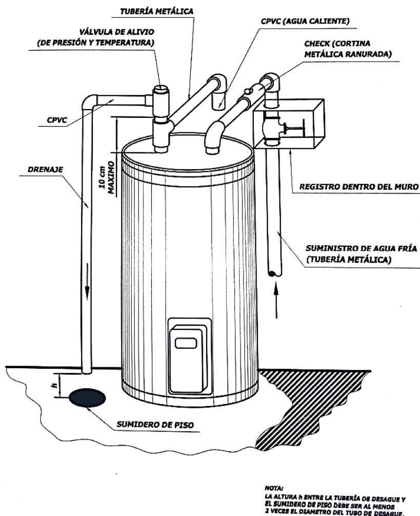
Figura 29. Esquema de calentador de agua Fuente: CIHSE, 2017
