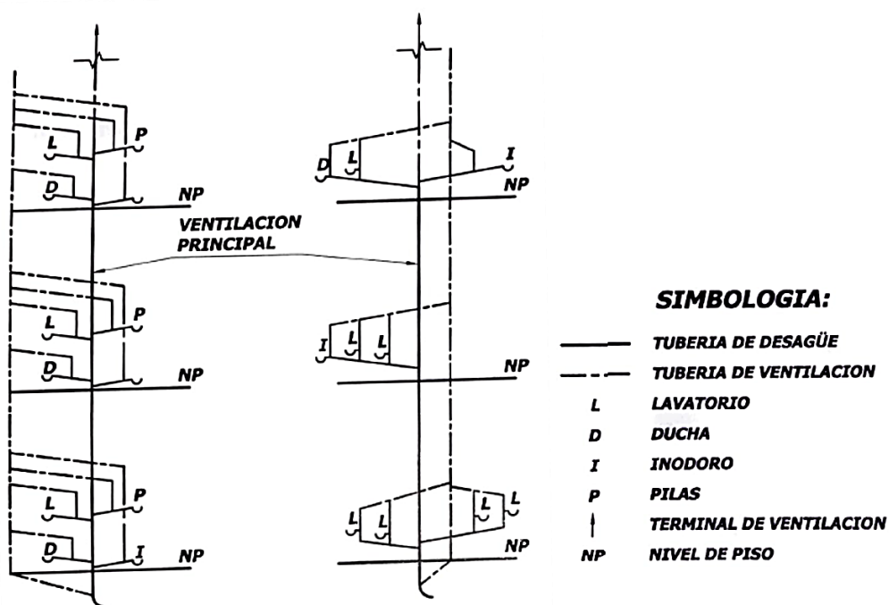
Figura 50. Sistema de ventilación individual Fuente: CIHSE, 2017
