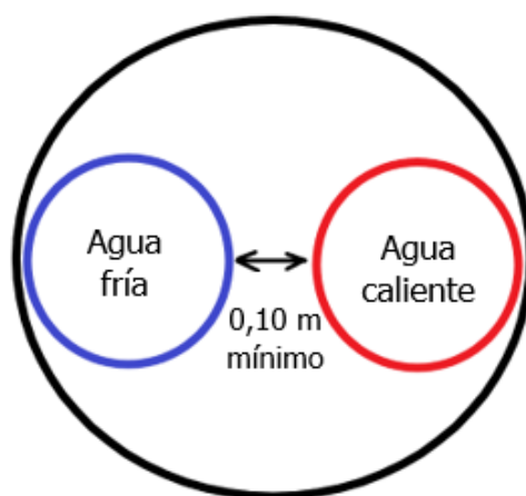
Figura 22. Distancia entre tubería de agua caliente y fría en un mismo ducto
