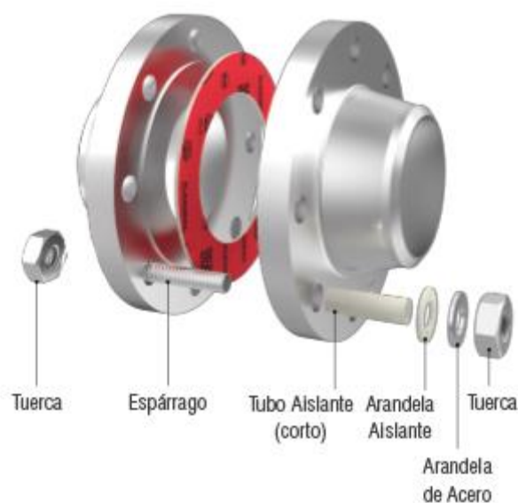
Figura 17. Kit de aislamiento simple para luminaria Fuente: Google, 2021
