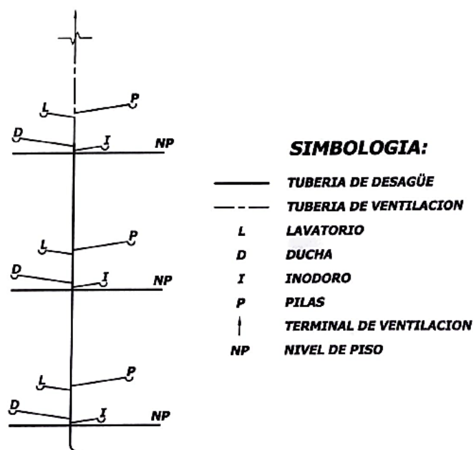
Figura 52. Sistema de ventilación de bajante único
