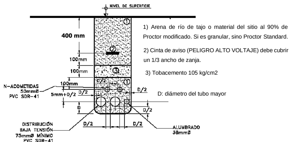
Figura 11. Esquema de acometida subterránea
