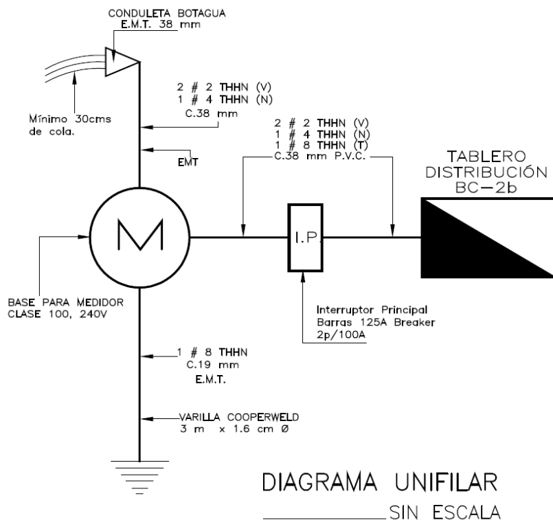
Figura 59. Ejemplo de diagrama unifilar Fuente: Google, 2021
