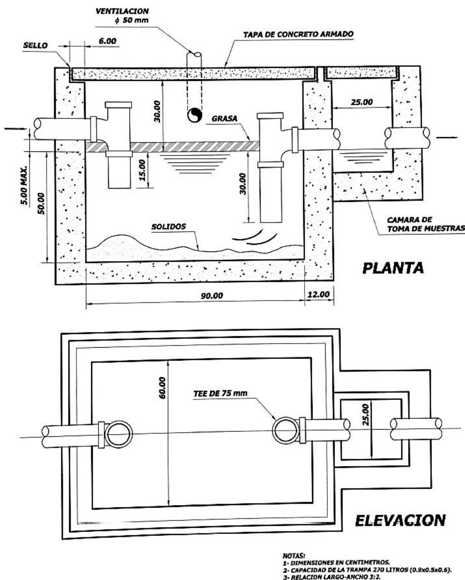
Figura 45. Trampa de grasa Fuente: CIHSE, 2017
