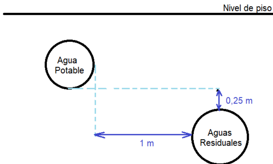
Figura 24. Distancia entre tuberías de agua potable y aguas residuales Fuente: Elaboración propia, 2021
