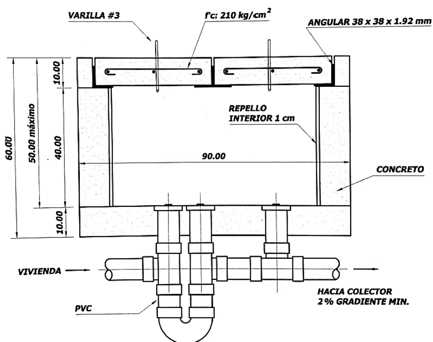
Figura 44. Sección B-B de caja de registro domiciliario con sifón Fuente: CIHSE, 2017
